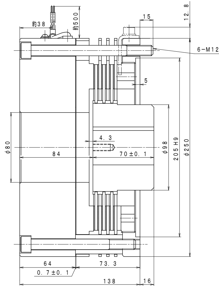
A—A' 断面
