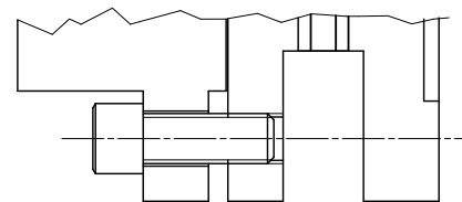
A-A' 断面図 (手動弛め取付時外觀)
