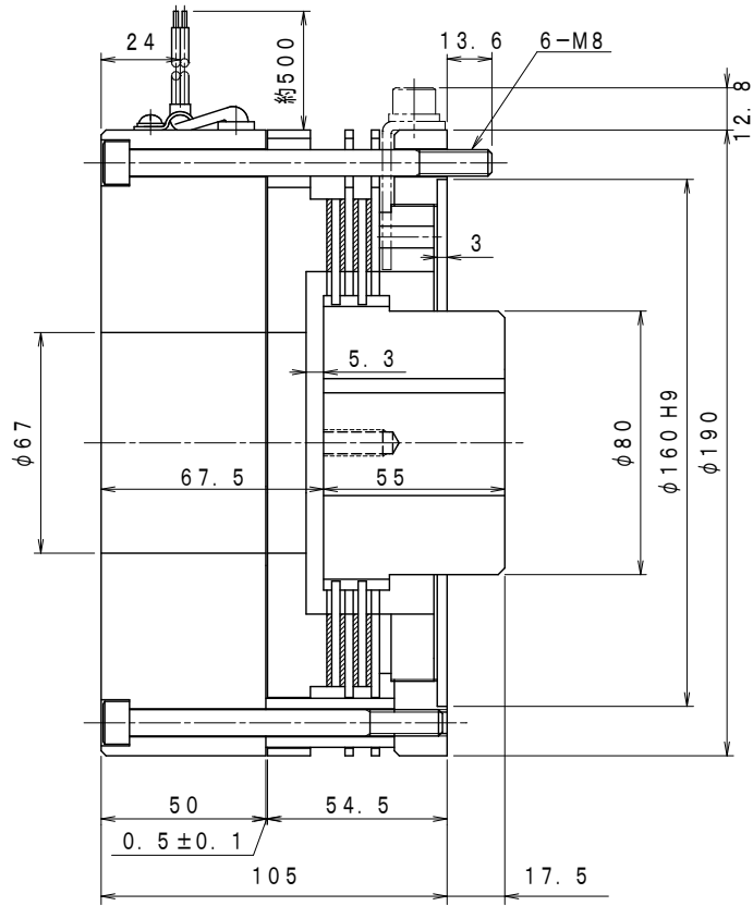
A-A' 断面
