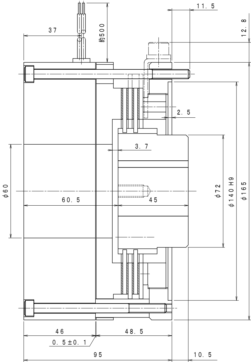
A-A' 断面
