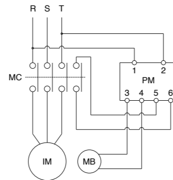
直流開閉
